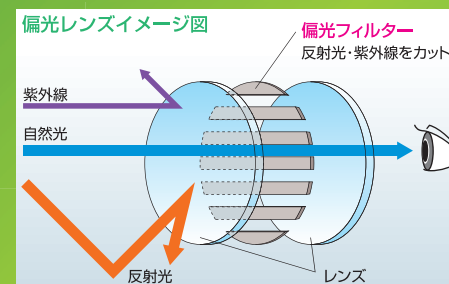
レンズの中に偏光フィルターを内蔵
